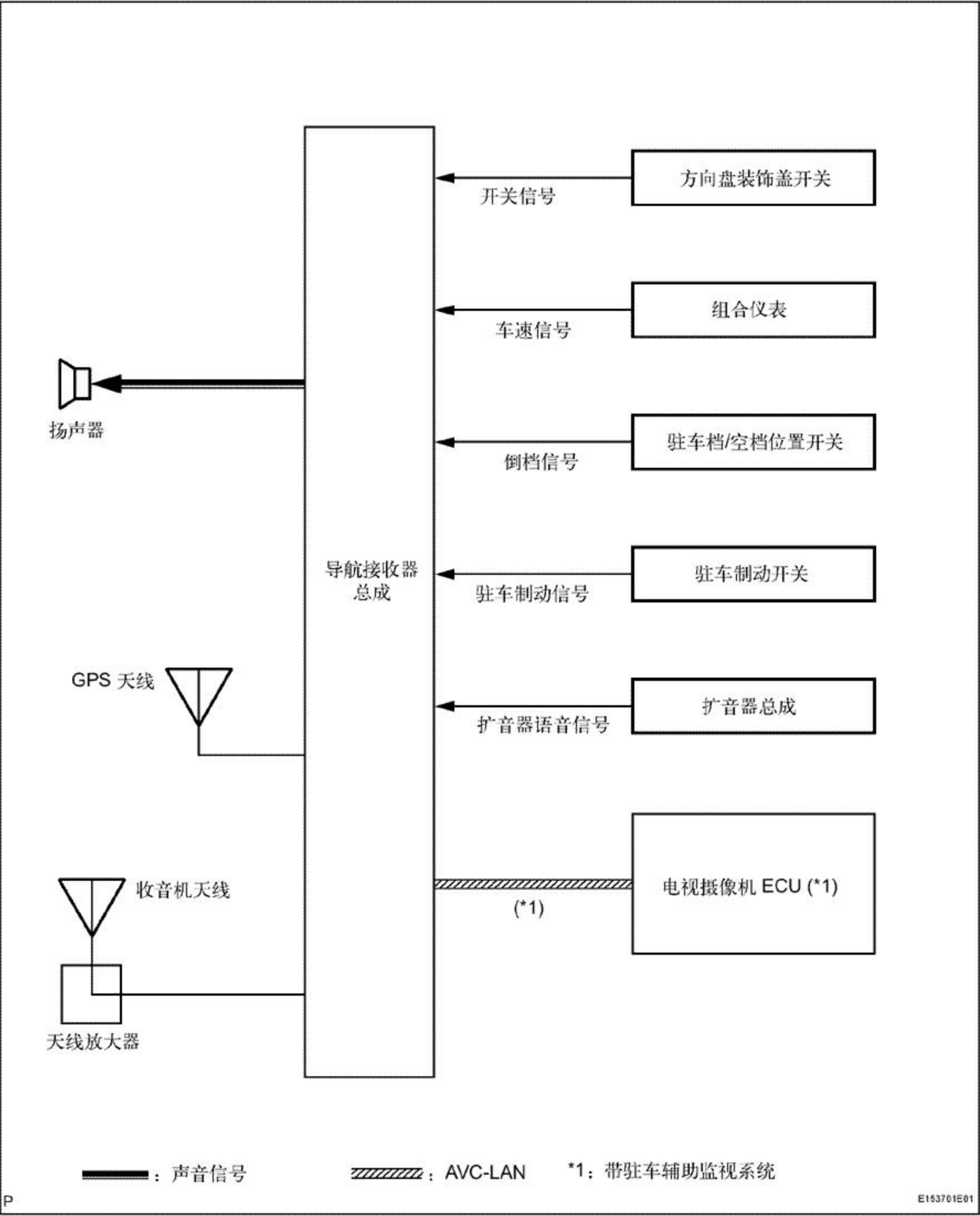
系统图
